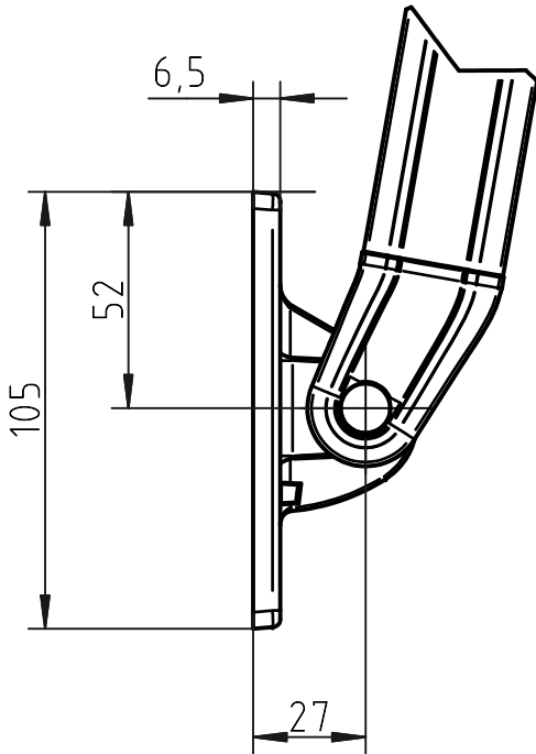
E ( 1 : 2 )
