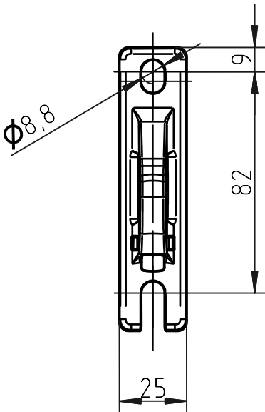
F ( 1 : 2 )
