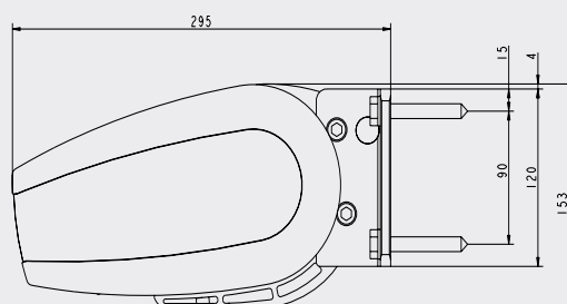
Sidovy FA64
